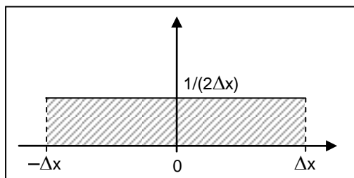
Loi uniforme sur [-\Delta x, \Delta x] L'aire de la surface hachurée est égale à 1.
